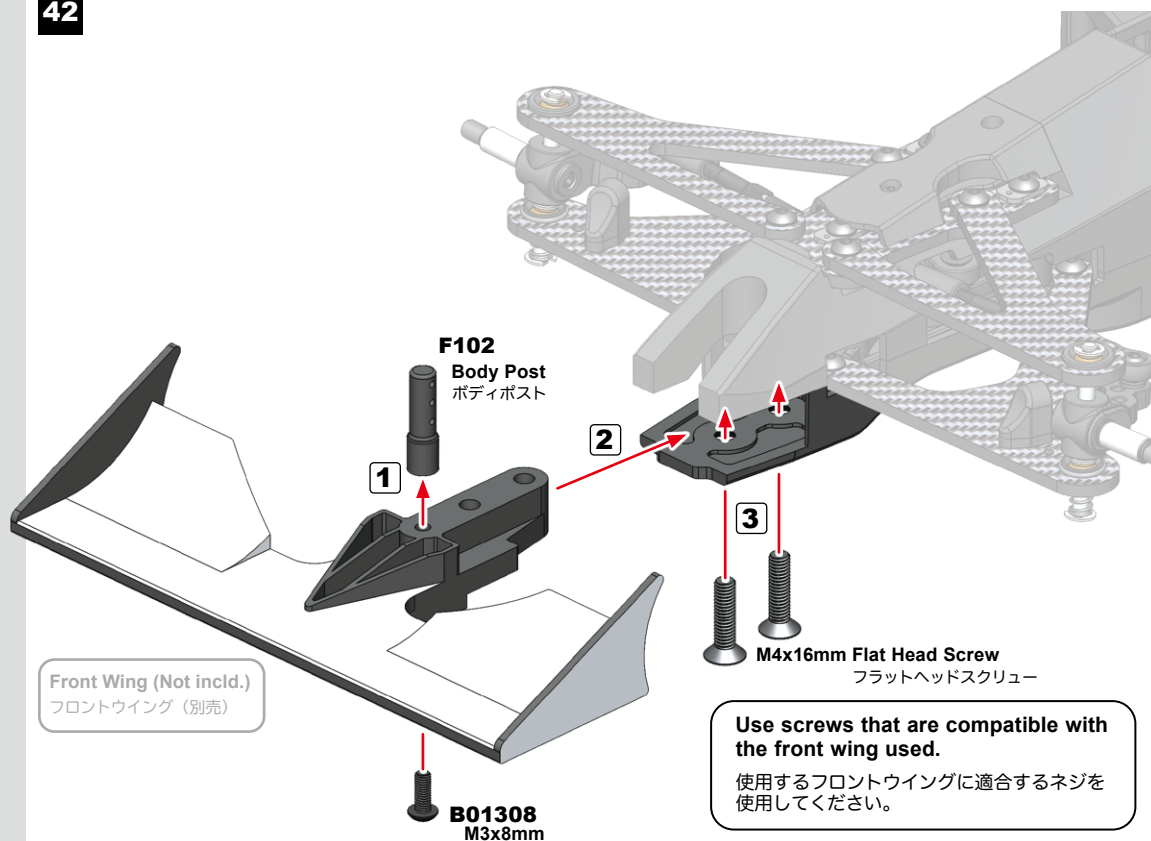
M4x16mm Flat Head Screw フラットヘッドスクリュー
