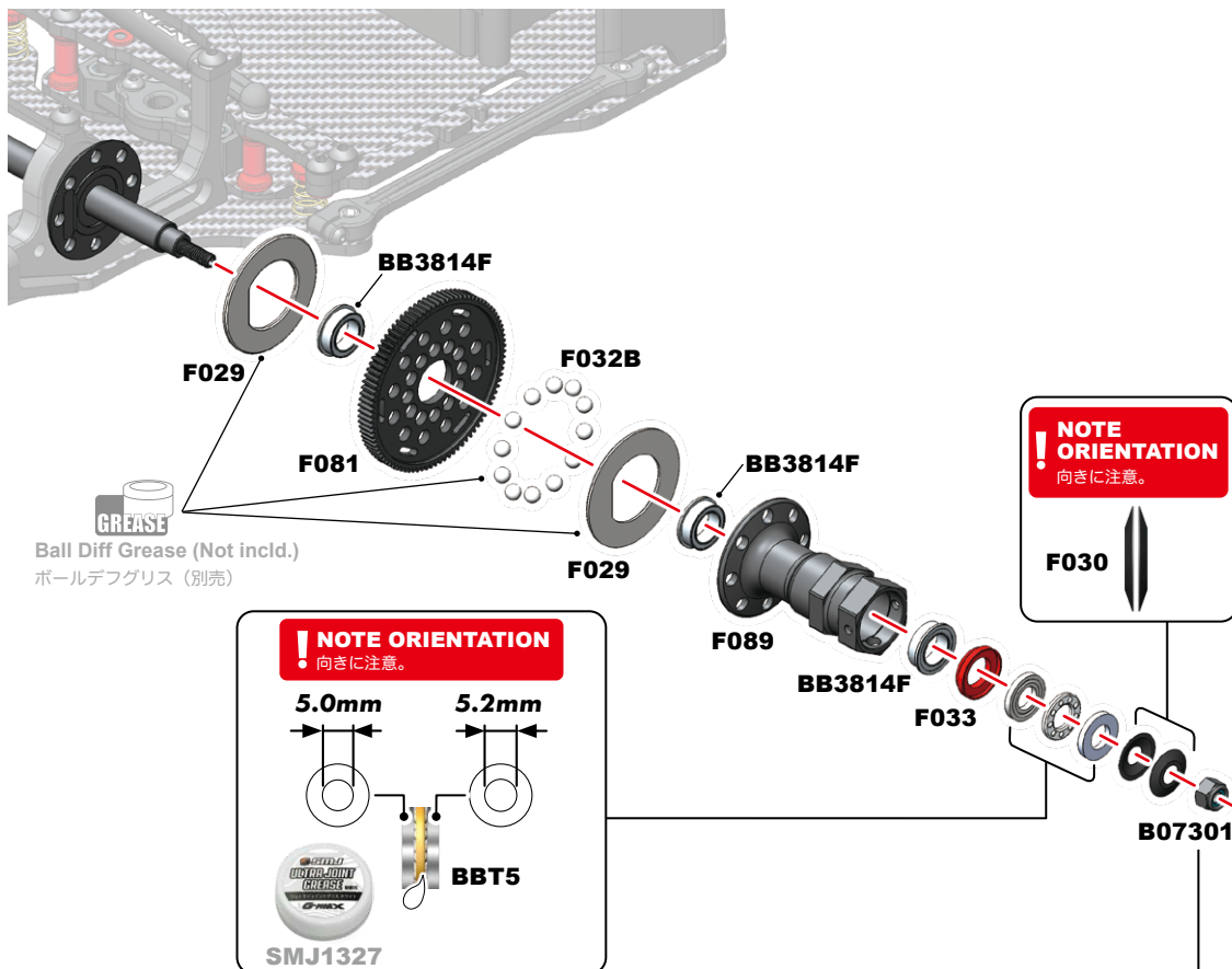
F033 x1 Alu Diff Thrust Bearing Washer アルミデフスラストベアリングワッシャー
