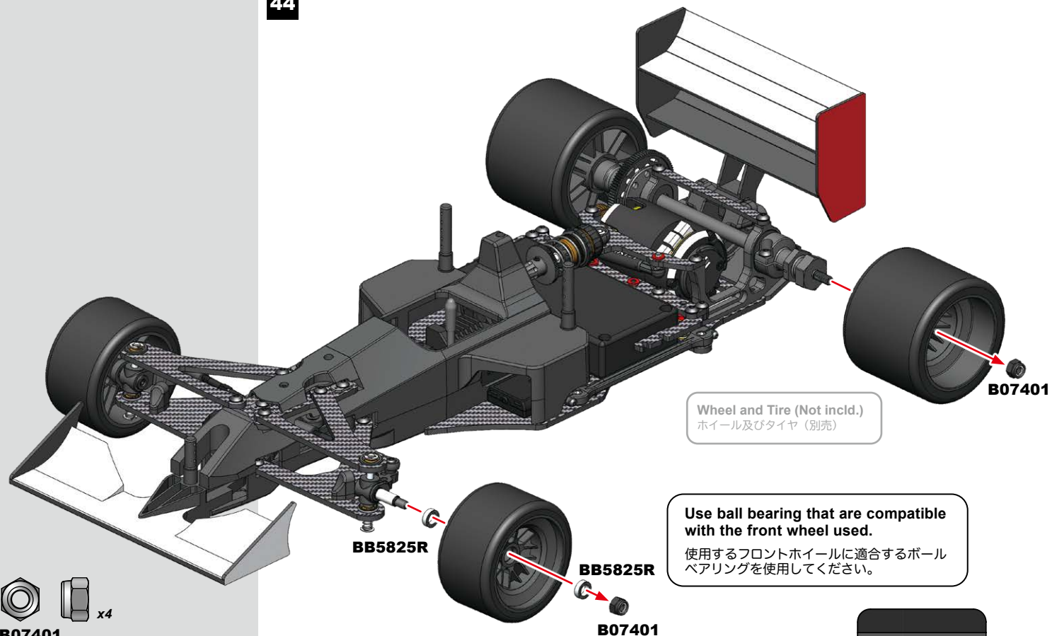
B07401 M4 Nylon Nut (Black) ナイロンナット (ブラック)
